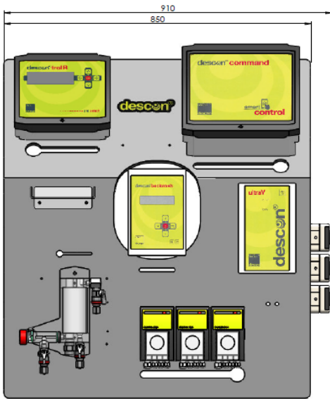
Montageeinheit / Vorbau PVC mit Geräteaufbau watercare complete 2.1
