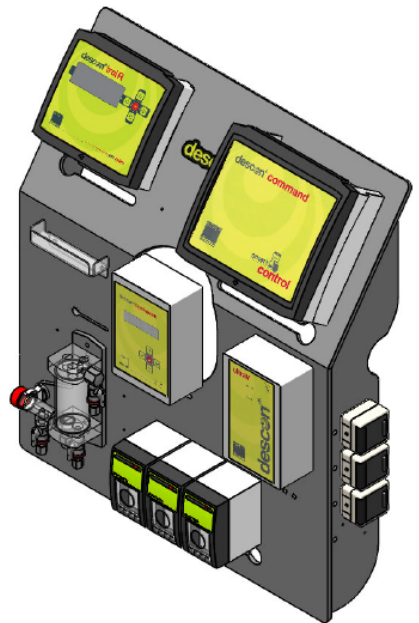
Montageeinheit / Vorbau PVC mit Geräteaufbau watercare complete 2.1
